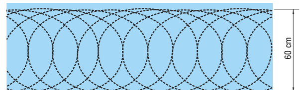
60 cm Yüksekliğinde Düzlemsel Jiletli Tel Flat Razor Wire - 60 cm Height Yükseklik Height : 60 cm Uzunluk Length : 10 cm
